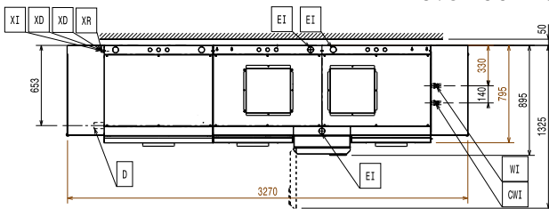
Boven aanzicht
